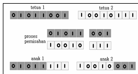
Gambar 1. Ilustrasi proses single point cross-over dalam GA.
